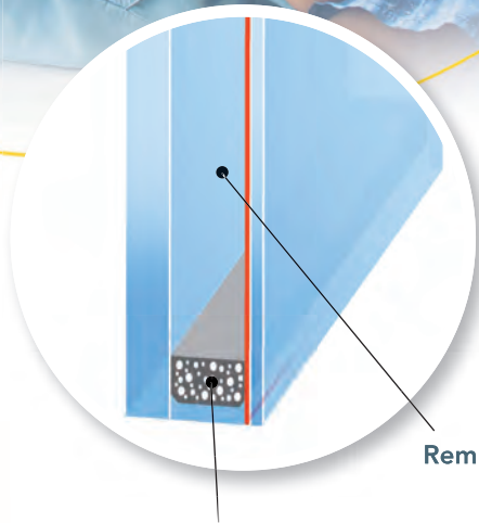
Intercalaire classique ou Warm edge
